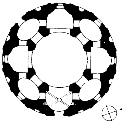
Kościół par. w Parkowie 1 : 500
